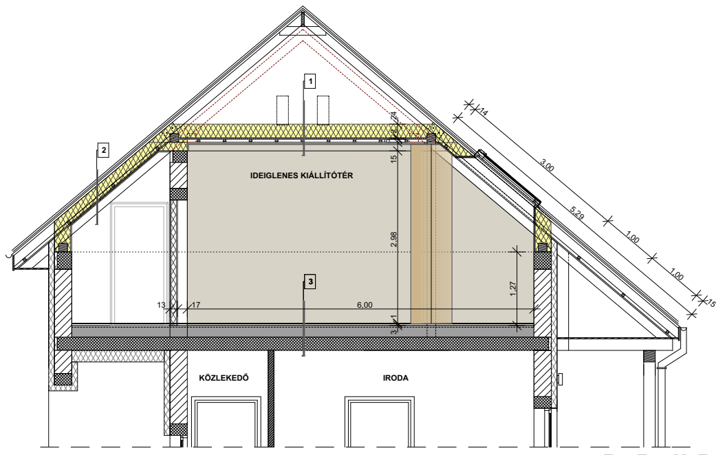
E-E METSZET
