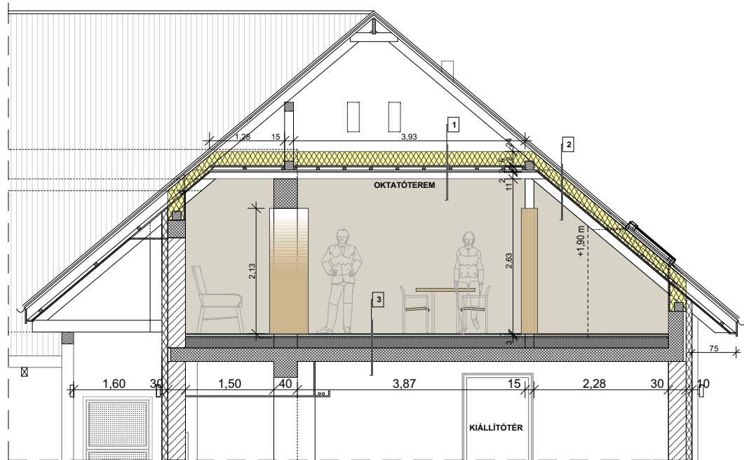
C-C METSZET
